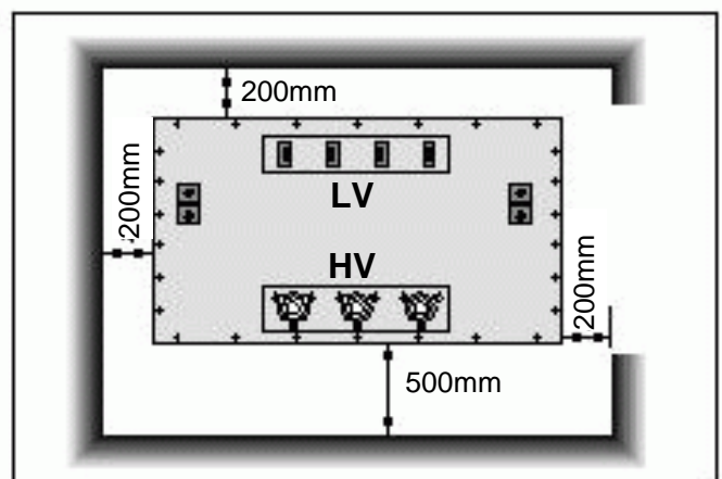
Hình 2 - Khoảng cách lắp đặt có vỏ bảo vệ IP20/21 Figure 2 – installation distance with enclosure IP20/21
