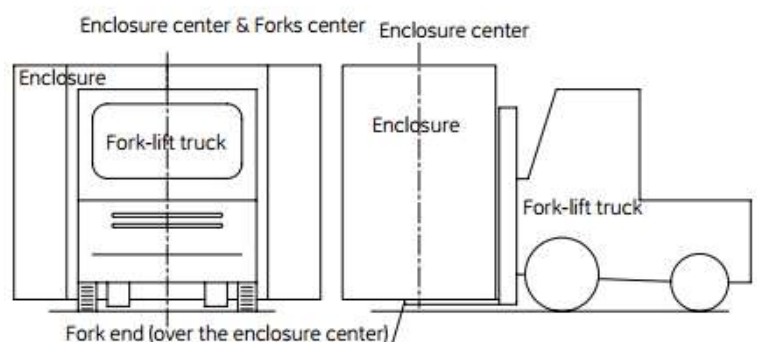
Hình 2. Nâng máy có vỏ tủ bằng xe nâng Transporting by fork-lift truck
